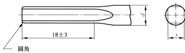
图4 B型:方形端部
