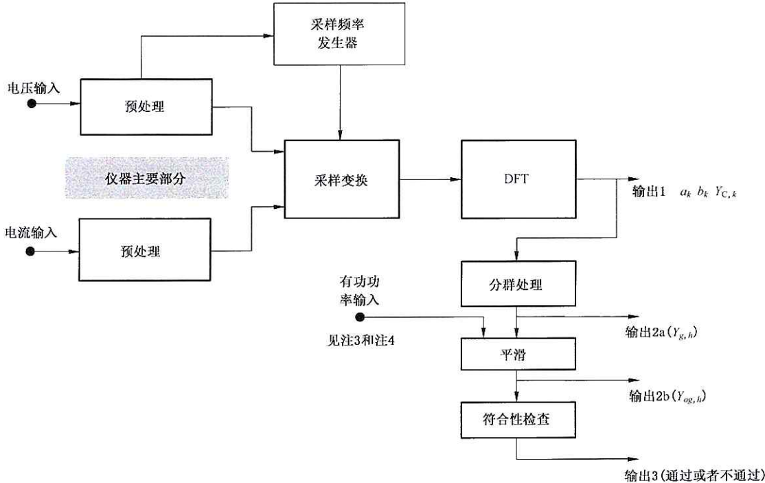
图 1 测量仪器的通用架构
