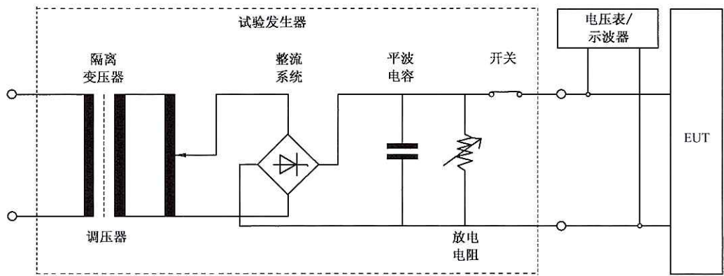
图 A. 1 以整流系统为基础的发生器示例
