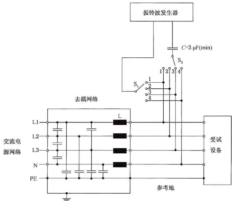
图 6 交/直流电源端口单相线对地试验
