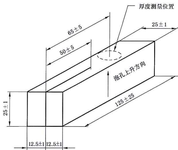
图 1 撕裂试样
